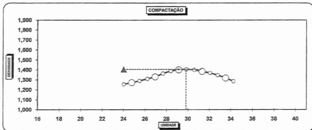
GRÁFICO DA CURVA DO ENSAIO DE COMPACTAÇÃO
