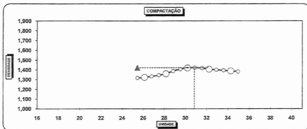
GRAFICO DA CURVA DO ENSAIO DE COMPACTAÇÃO
